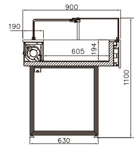
VMINCPPDASP-VDB UV padaria c/ sistema de aspiração bakery w/ vacuum system
