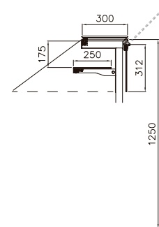
OPÇÃO: VDA CH c/ sistema hidráulico de abertura w/ lift-up opening system
