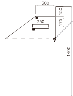
OPÇÃO: VDA SH vidro de rebater tilt-down opening
