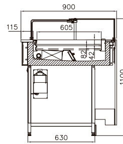
VMINVSCHR-VDB UV 3M2 ventilada c/ sistema de humificação ventilated w/ humidification system
