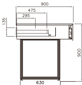
CX1N MIN caixa de saída support counter
