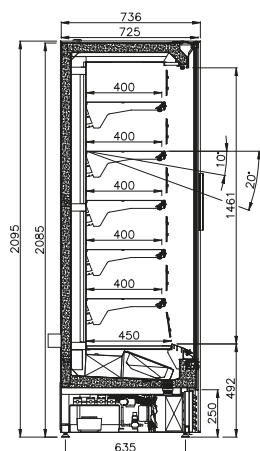
Sección refrigerada -1...+5 °C (3M1)
