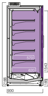
MF2 900 N CP SG 3L1 congelados frozen food
