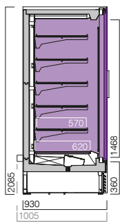
MF2 900 N CP CG 3L1 congelados frozen food
