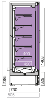
MF2 700 N CP CG 3L1 congelados frozen food
