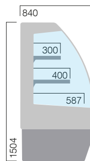
SMVCT 3N H15 3M2 refrigerado ventilado chilled ventilated +3°... +6° C dim. 625 | 937 | 1250 | 1875
